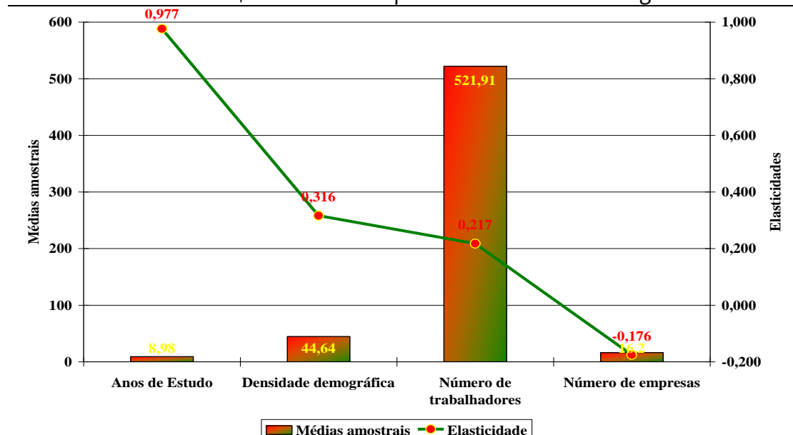
Figura 3. Elasticidade renda em relação a anos de estudo, número de trabalhadores, número de empresas e densidade demográfica
