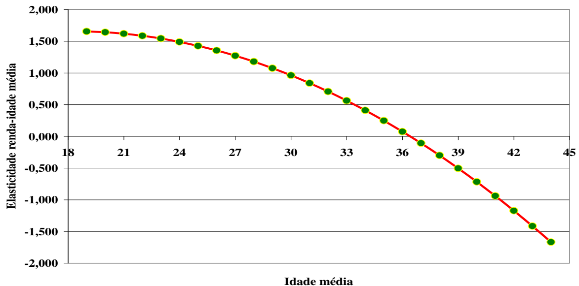
Figura 4 Variação da elasticidade renda idade média entre os 19 e 44 anos dos trabalhadores da Indústria de máquinas e implementos agrícolas no Noroeste do Rio Grande do Sul
