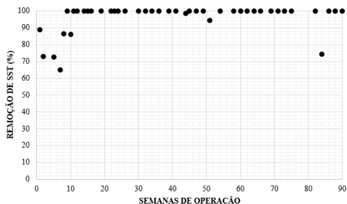
Figura 2 – Eficiências de remoção de SST do wetland construído vertical de fundo saturado.
