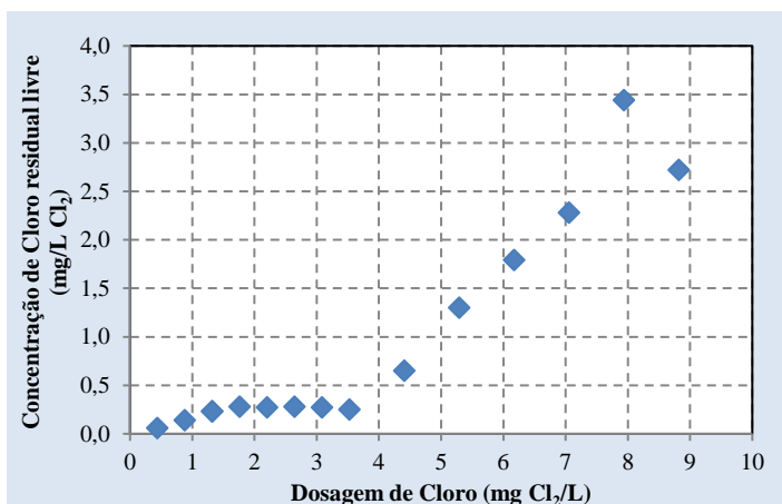
Figura 3 – Resultados do ensaio de demanda de cloro da água de reuso coagulada com PAC.
