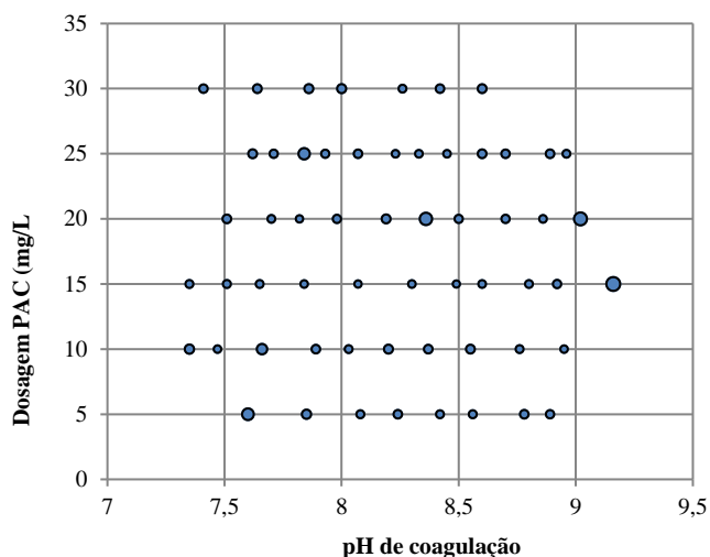
Figura 2 – Ensaio em jar-test simulando FDD para construção do diagrama de coagulação e otimização da dosagem de PAC, através da turbidez remanescente.
